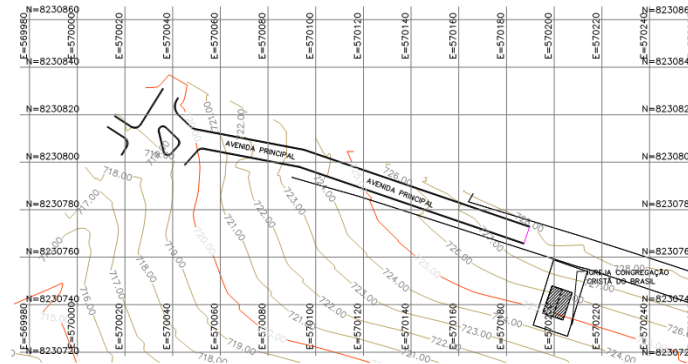
1 PLANTA PLANIMÉTRICA ESCALA 1:1000
