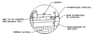
03 DETALHE DA SERJETA E DO MEIO FIO/ CORTE PADRÃO ESCALA 1:20
